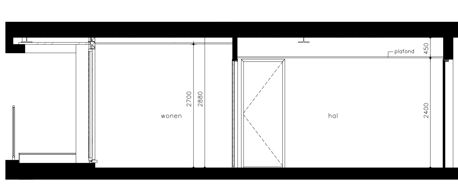
Doorsnede
